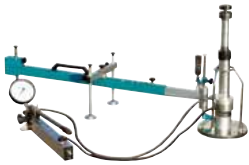
10-2350 Plattendruckgerät 100 kN Plate Bearing Test Set 100 kN
